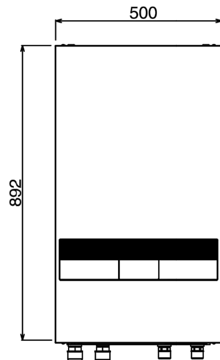
FRONTANSICHT
