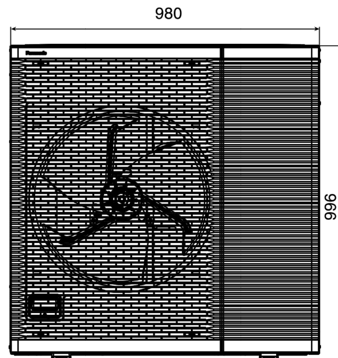
Vorderansicht
