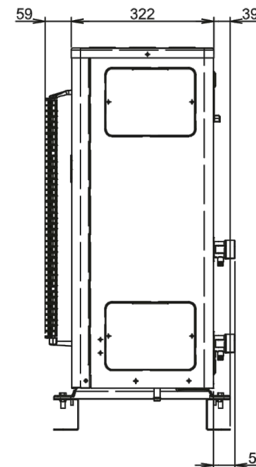
Seitenansicht rechts
