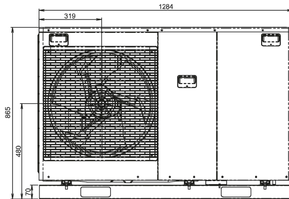
Frontansicht
