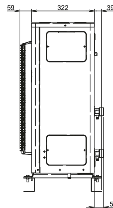
Seitenansicht rechts
