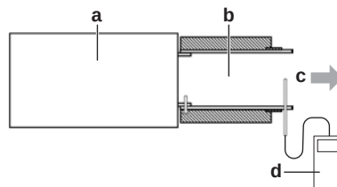
a SV-Einheit b Luftauslass-Kanal c Luftstromrichtung d Hitzdrahtanemometer
