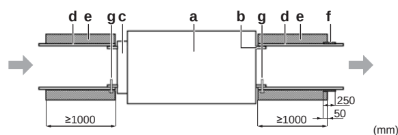
a SV-Einheit
