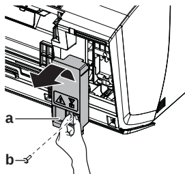
a Wartungsblende
