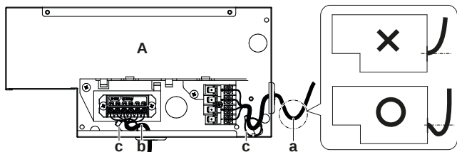
A Inneneinheit-Platine(ASSY) a Verkabelung der Stromversorgung und Erdung b Anschluss des Übertragungs- und Benutzerschnittstellenkabels c Rohrschellen X Nicht zulässig O Zulässig
