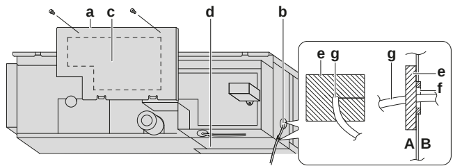
A Außerhalb des Geräts B Innerhalb des Geräts a Steuerkastenabdeckung b Anschluss des Verbindungskabels (einschließlich Erde) c Schaltplan d Anschluss des Benutzerschnittstellenkabels e Dichtungsmaterial (Zubehör) f Kabelöffnung g Draht
