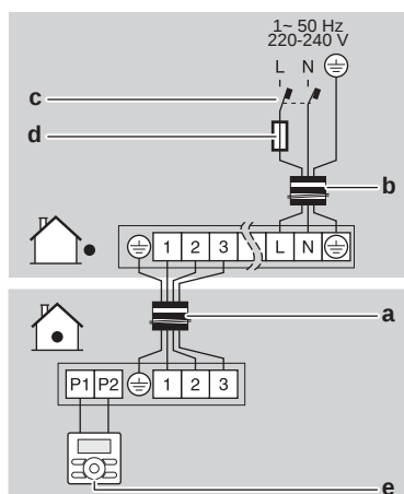
a Verbindungskabel b Stromversorgungskabel
