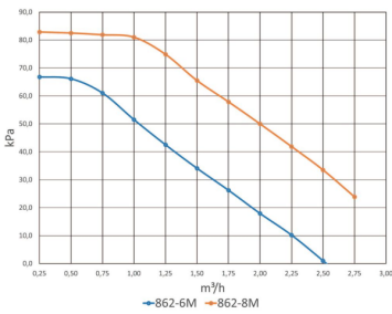
LK 862 - PUMPENCHARAKTERISTIK
