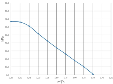
LK 866 & LK 867 - PUMPENCHARAKTERISTIK
