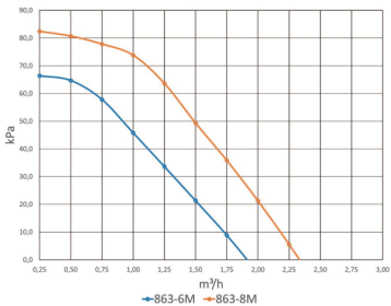
LK 863 - PUMPENCHARAKTERISTIK
