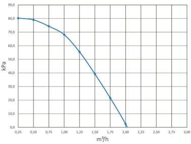
LK 865 - PUMPENCHARAKTERISTIK
