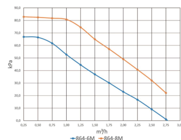
LK 864 - PUMPENCHARAKTERISTIK
