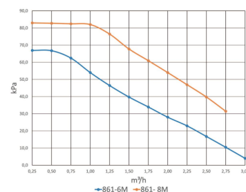
LK 861 - PUMPENCHARAKTERISTIK
