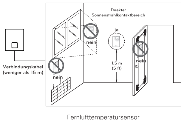
Fernlufttemperatursensor
