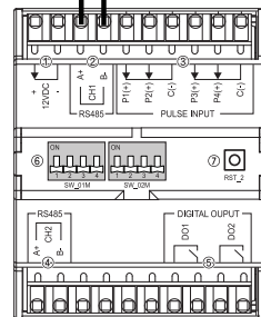
Zählerschnittstelle
