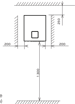
Mindest -Wartungsabstände (Gerät: mm)
