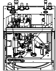
Verkabelung für „KOMBIKOMBINATION-2“
