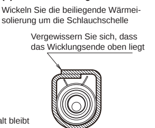
(d) Schlauchöffnungs-Ansicht
