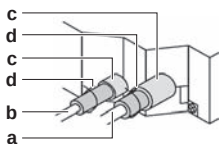
Abb. 4.3: Isolieren der Wasserrohrleitungen
