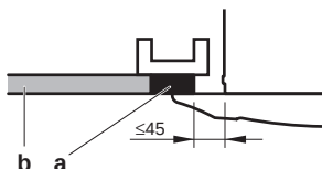
Abb. 4.1: Platz in der Decke zu groß
