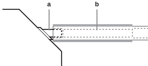
Abb. 4.6: Anschließen der Abflussleitung
