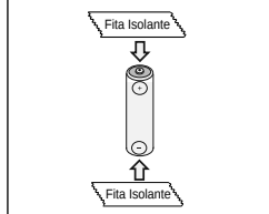
Fig. 1 Como isolar os terminais
