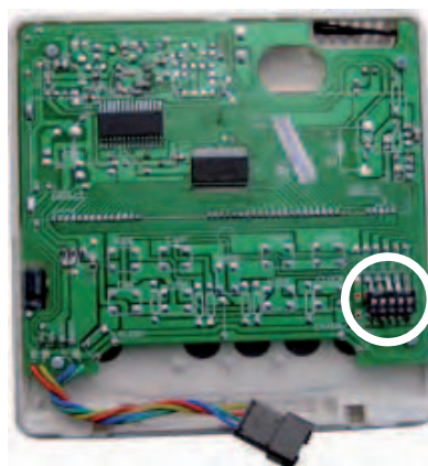
Dipschalter
