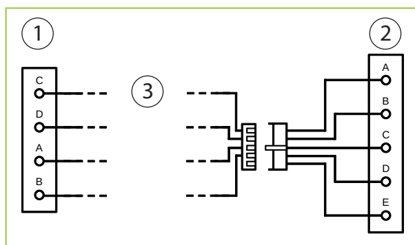
Abb. 4: Elektrisches Anschlussschema
