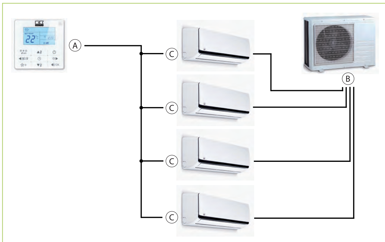
Abb. 7: Montage Multisplitkombination mit einer Fernbedienung
