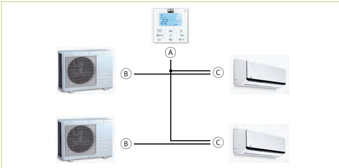
Abb. 6: Montage zweier Singlesplitkombinationen mit einer Fernbedienung
