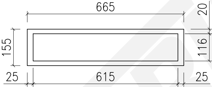
US 665x155-615x116
