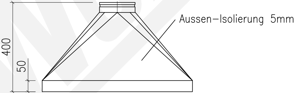
Steckverbinder DN160
