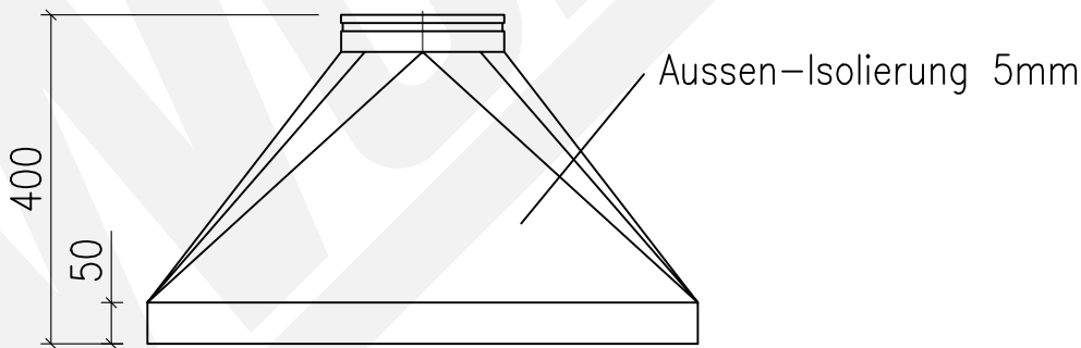
Steckverbinder DN200
