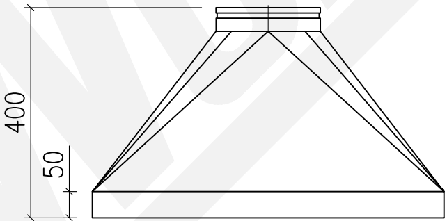
Steckverbinder DN200
